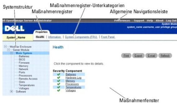
Abbildung 3-2. Beispielstartseite von Server Administrator - modulares System
